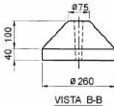
ANCLA CÓNICA C1
