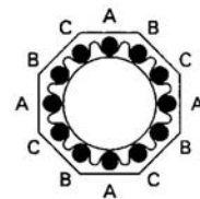
Localización de las varillas sección de los postes CR-12E.
